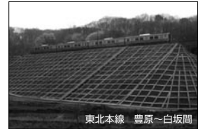
盛土の面工(吹付砕工)
