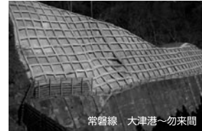
自然斜面防護工(吹付砕工)
