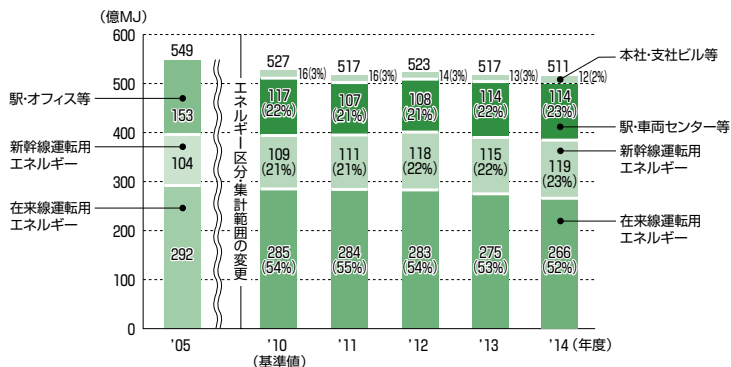
○ JR 東日本 消費エネルギーの構成
