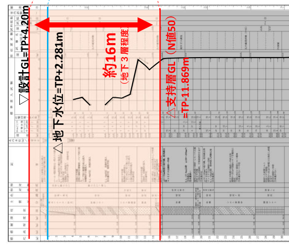
5街区建物付近地質柱状図
