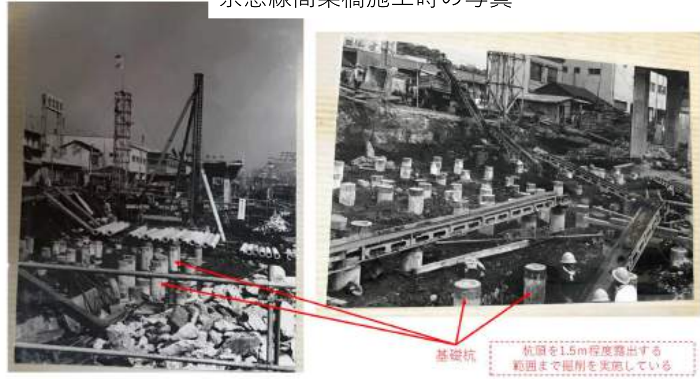
京急線高架橋施工時の写真
