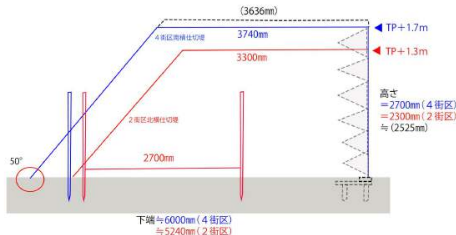
【南横仕切堤南面(4街区)】
