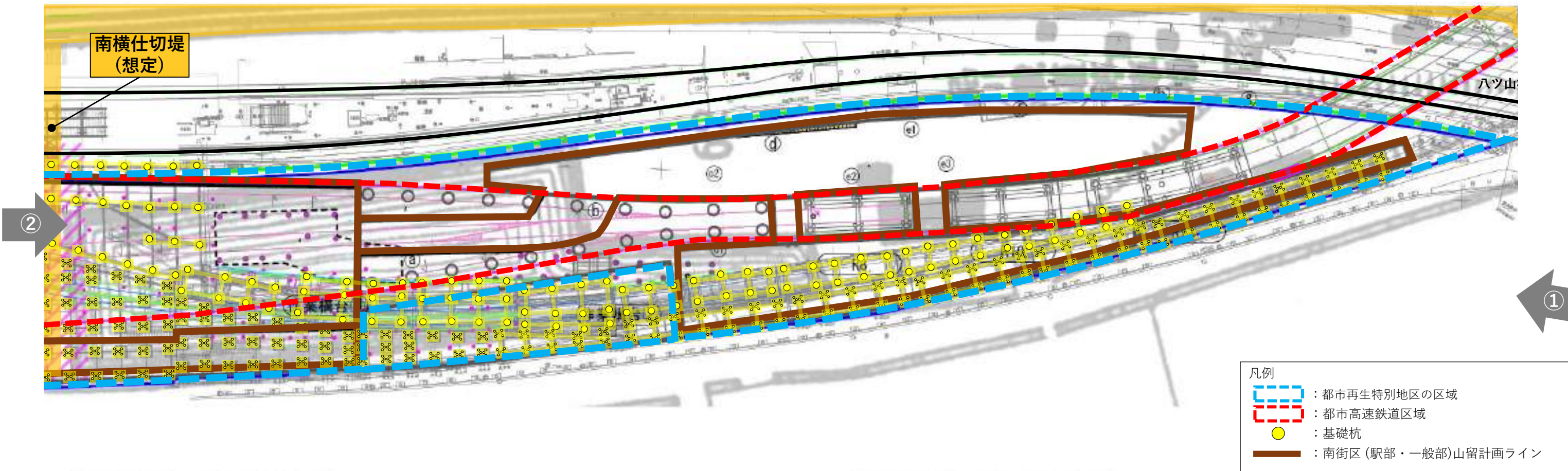
①品川駅以南の現況【2023年頃】
