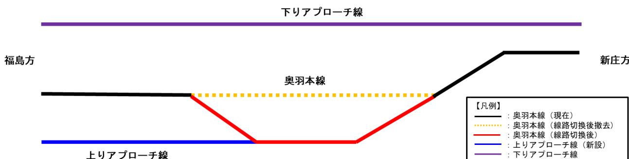
【今回工事範囲拡大 線路切換概要図】
