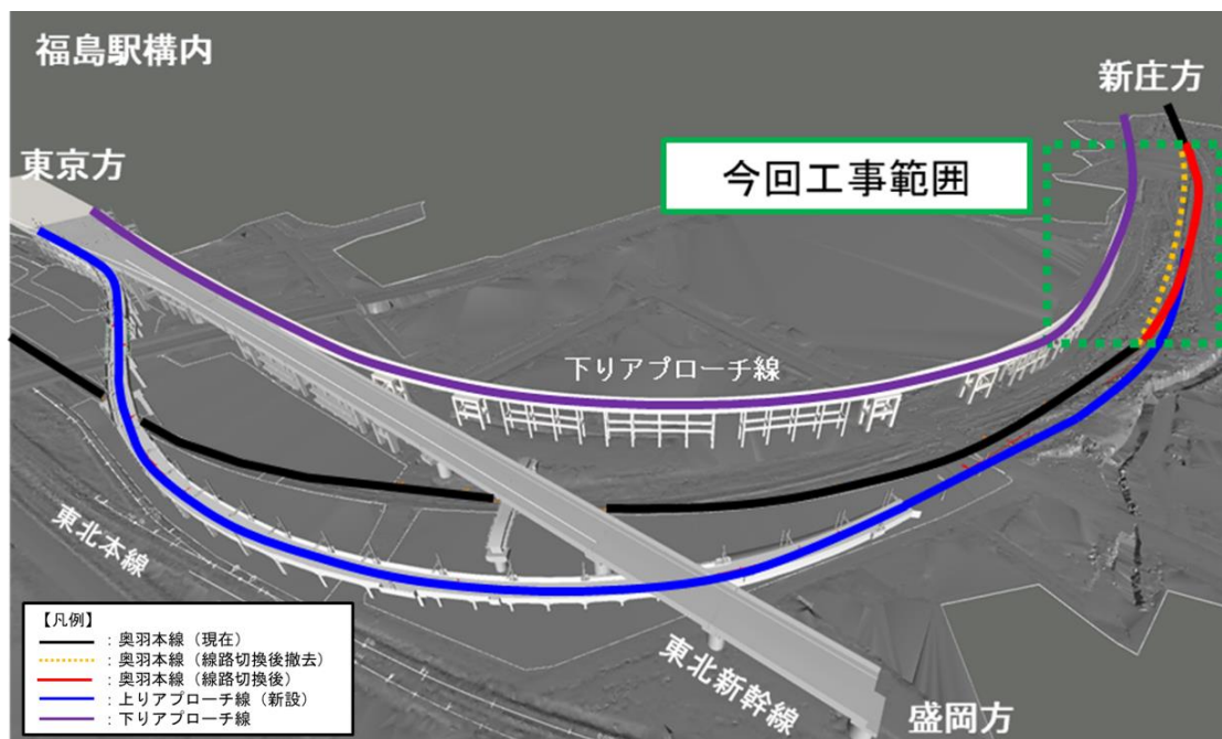
【奥羽本線 線路切換 全体イメージ図】
