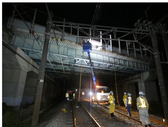
立体交差箇所の点検イメージ
