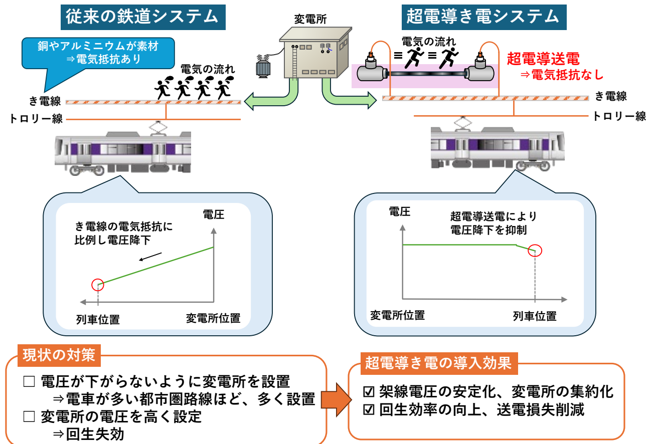
図2 超電導き電システムの概要
