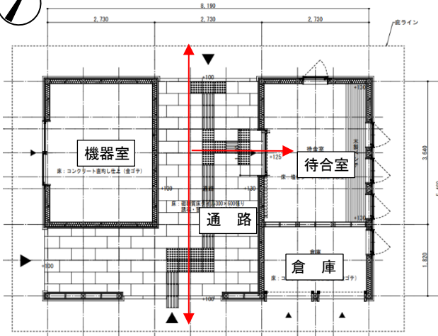
【新駅舎 平面図】
