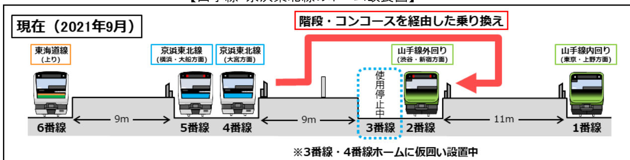
【山手線・京浜東北線のホーム改良図】
