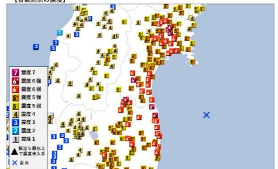
【各観測点の震度】
