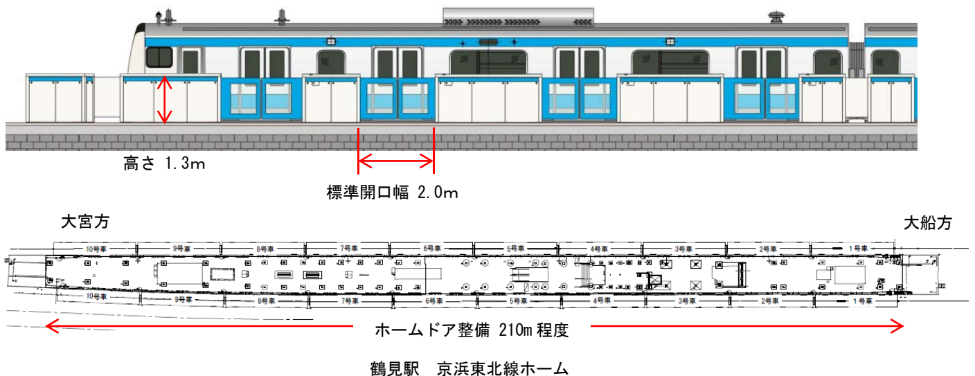
ホームドア設置イメージ
