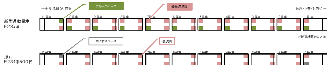
優先席・フリースペース配置イメージ
