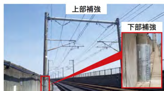
電柱耐震補強
