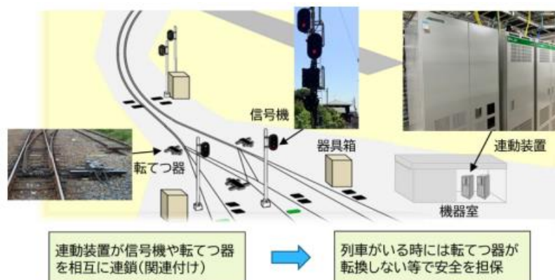
図-2 連動装置
