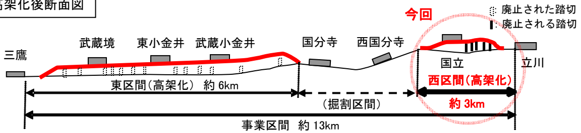
高架化後断面図
