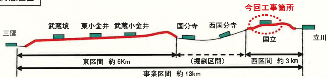
現状断面図
