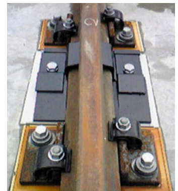
レール転倒防止装置
