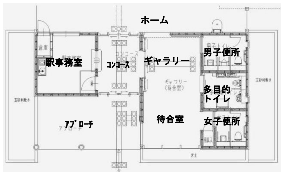
新駅舎平面図
