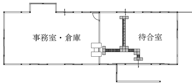
駅舎 平面図
