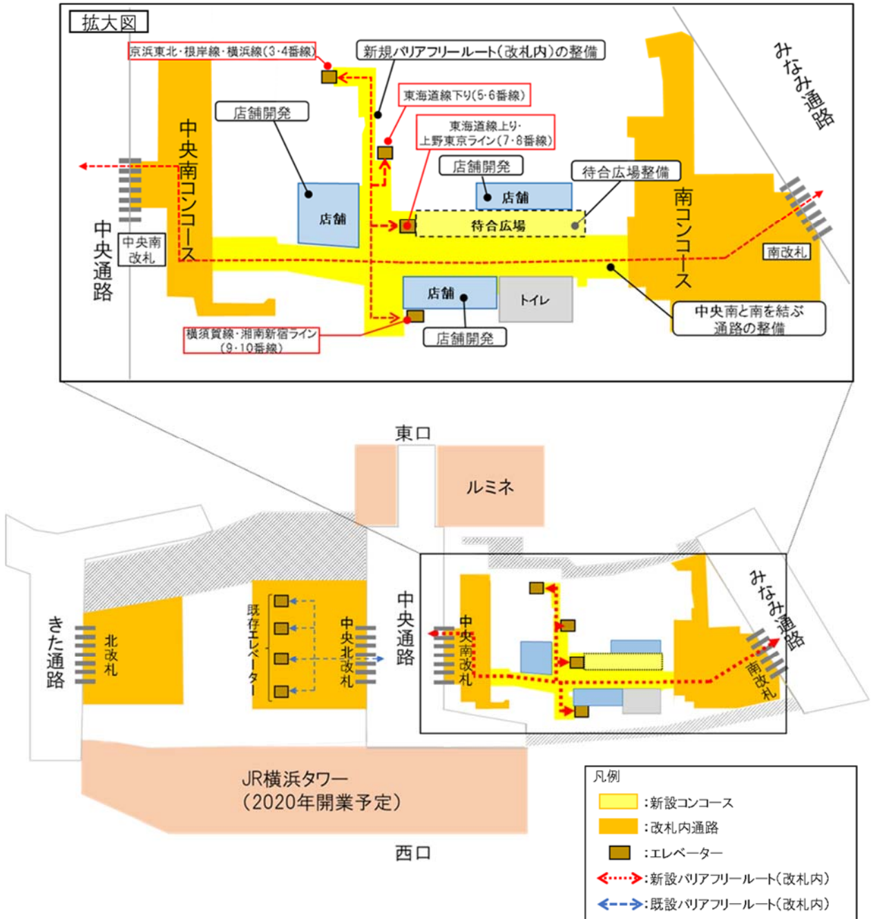
【参考図】 JR 横浜駅 整備計画概略図
