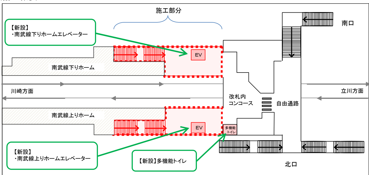
改札内バリアフリー設備 平面図
